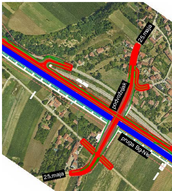
Podvožnjak 4 na km 197+385.00
