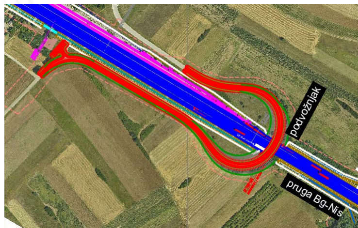
Podvožnjak 7 na km 205+802.81
