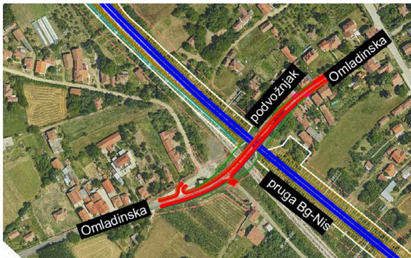
Podvožnjak 6 na km 202+340.10
