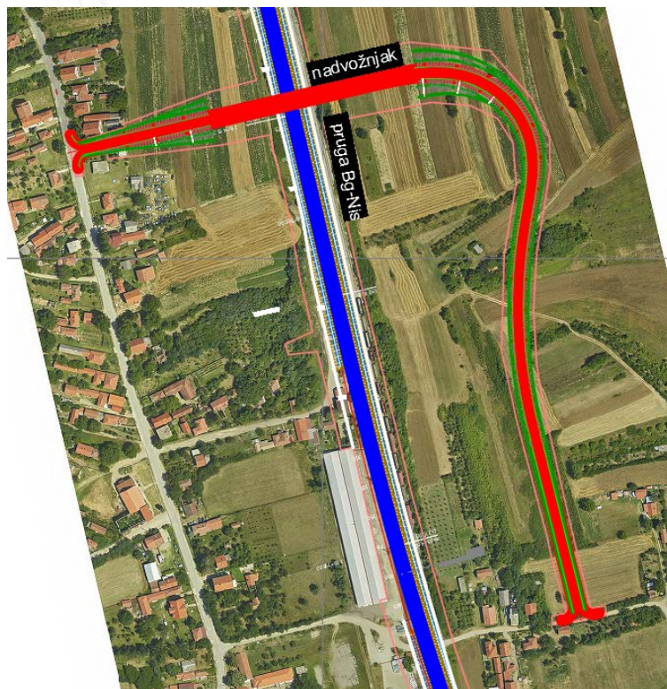
Nadvožnjak 14 na km 219+404.73
