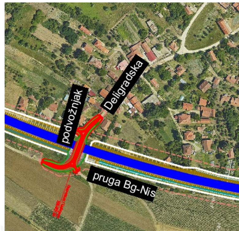
Podvožnjak 8 na km 206+821.81
