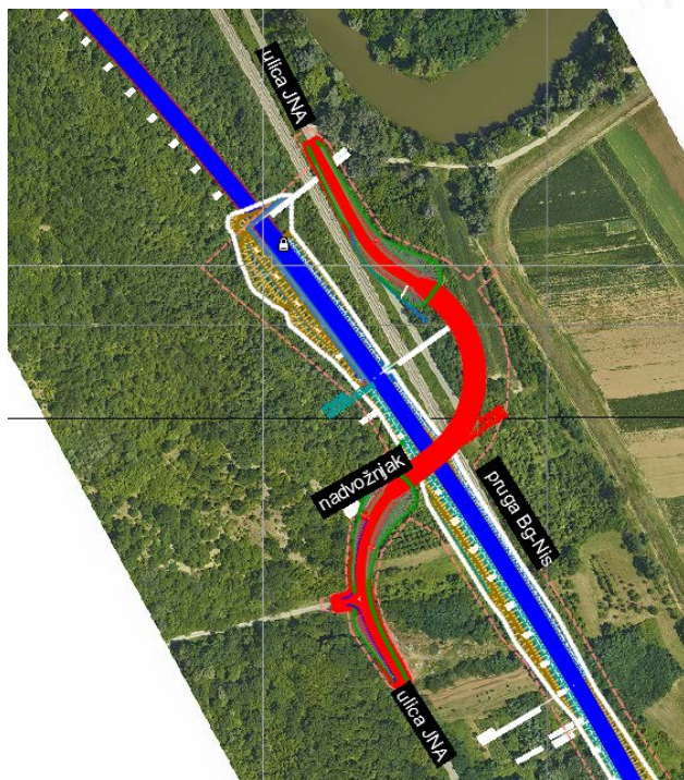
Nadvožnjak 1 na km 193+053.51
