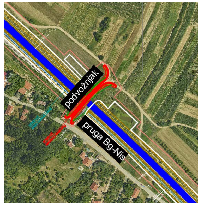
Podvožnjak 15 na km 221+359.49
