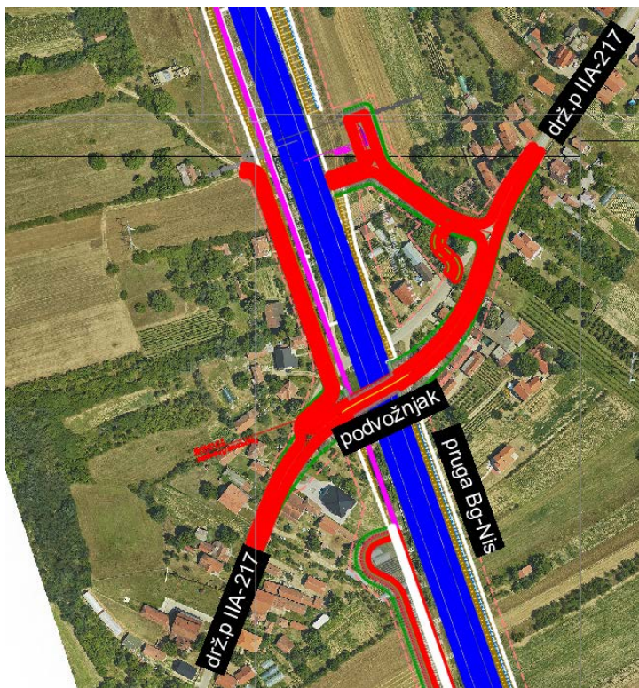
Podvožnjak 13 na km 217+044.39
