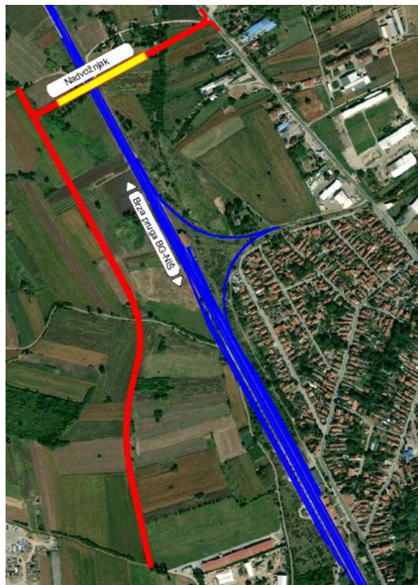
Nadvožnjak 1 na km 153+941.53
