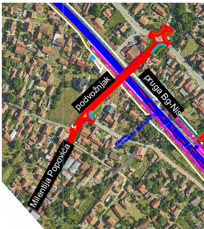
Podvožnjak 9 na km 208+744.21
