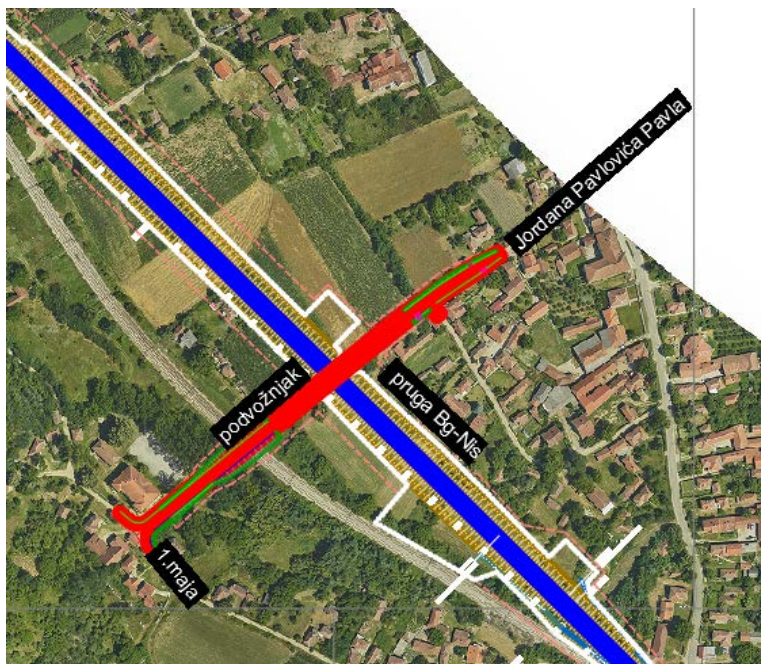
Podvožnjak 3 na km 196+165.06
